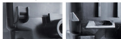
Vecchio aggancio riscaldatore Old hooking heater Nuovo aggancio riscaldatore New hooking heater
